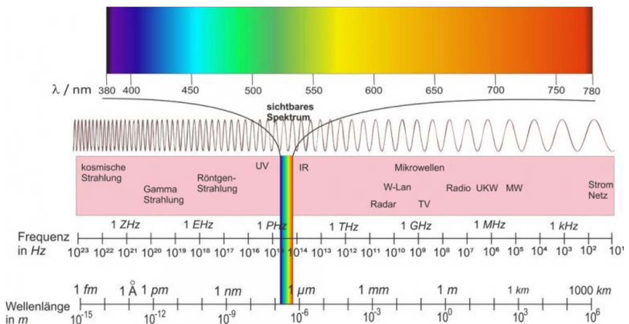
Abbildung 3.4-1: Der Wellenlängenbereich der optischen Strahlung.
